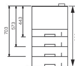
◎正面図
