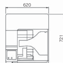
◎上面図
